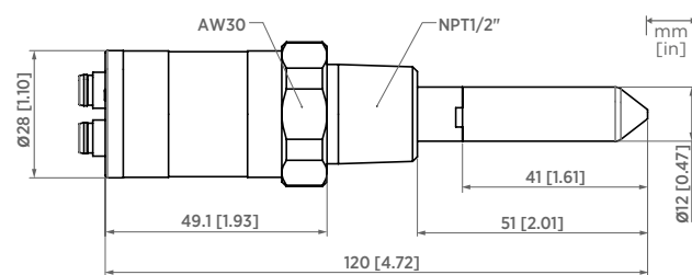
NPT1/2"ネジ付き DMT143L
