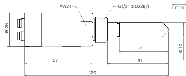
G1/2"ネジ付き DMT143L
