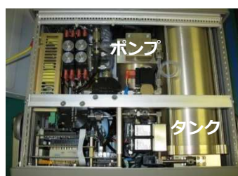
MBW973-SF6 内部写真
